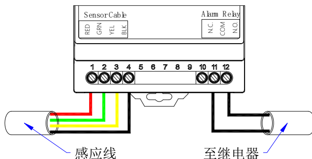
图 6 感应线与继电器连接示意图
