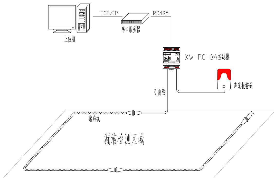
图 3 系统拓扑图
