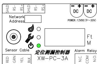
图 7 接电面板示意图
