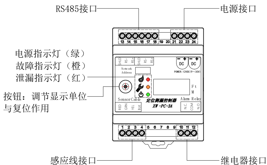
图 2 指示灯、按钮与端口说明示意图
