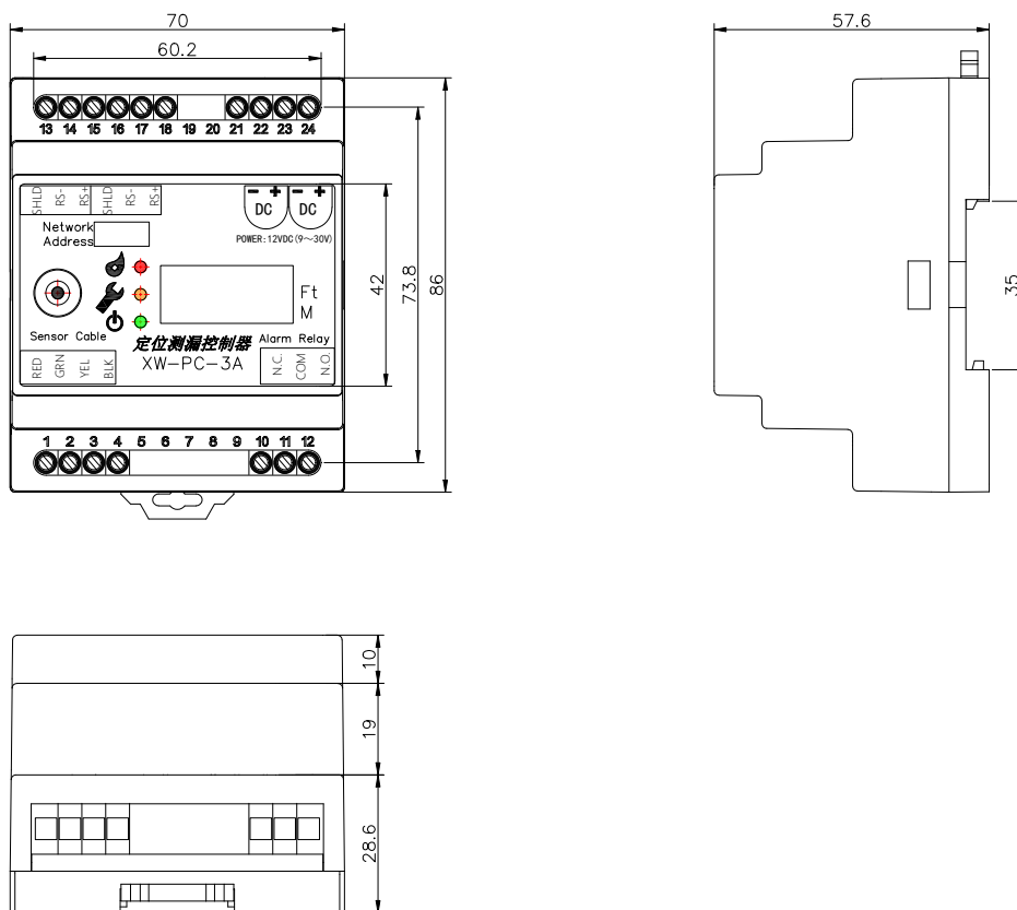
图 1 尺寸图
