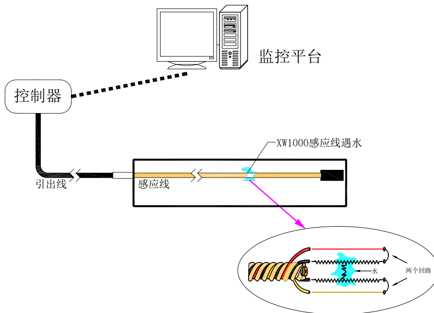
图 1 原理示意图
