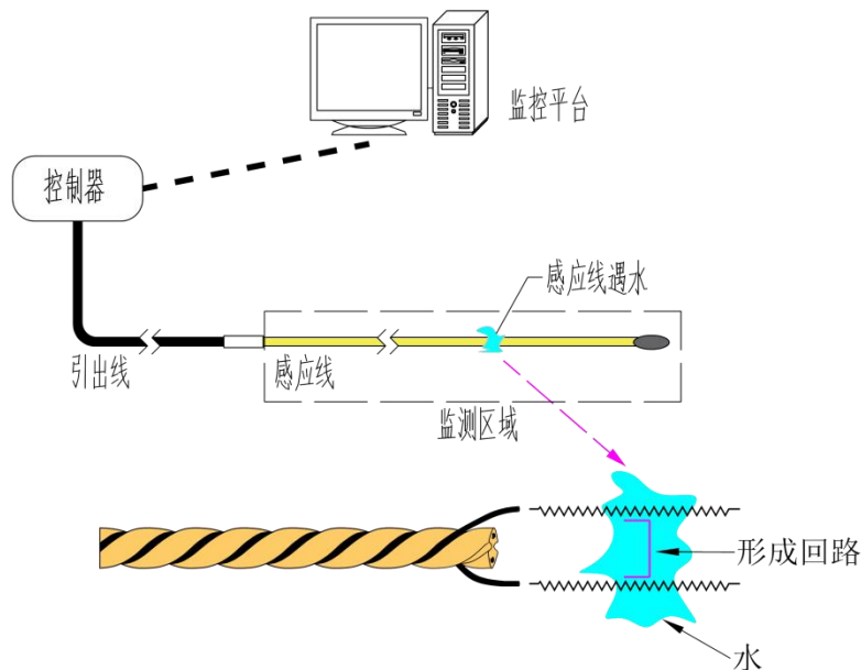
图 1 原理示意图
