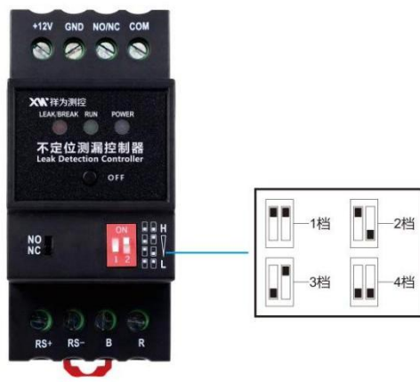
图 4 灵敏度档位按键调节示意图
