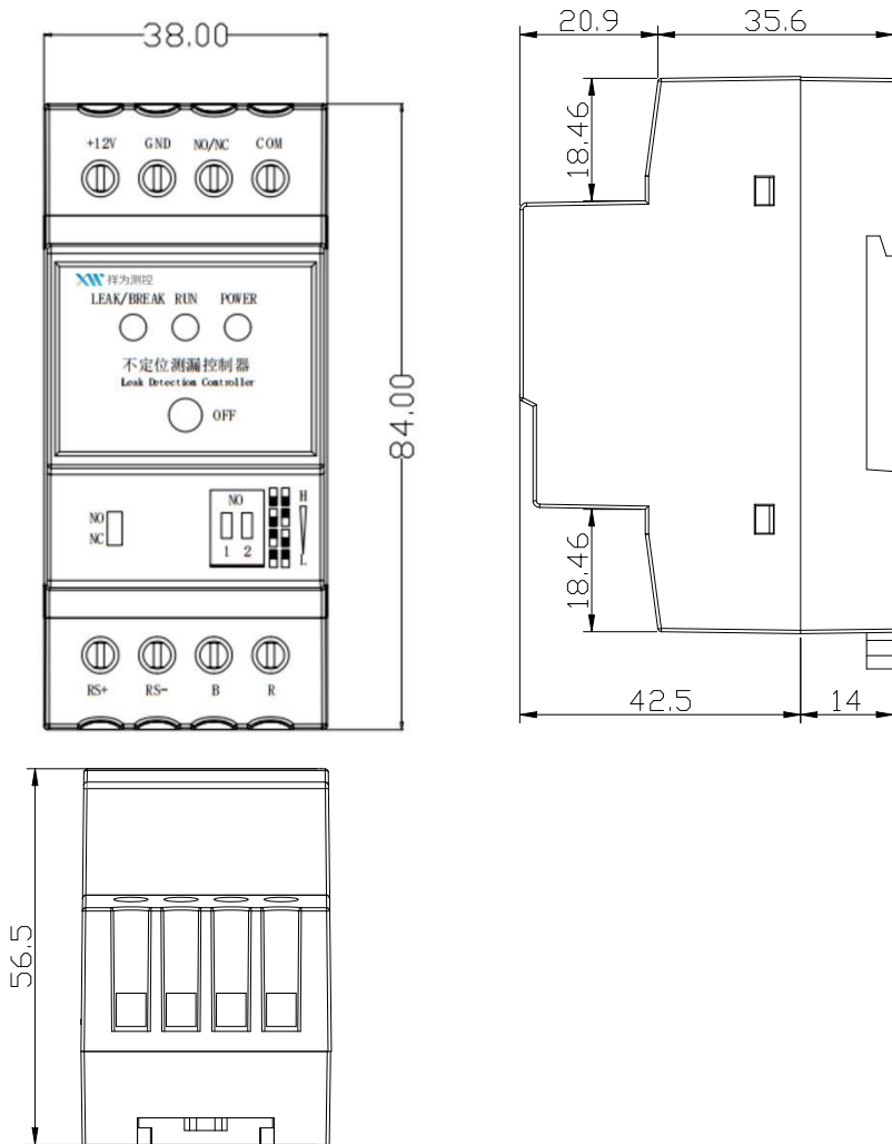
图 2 控制器尺寸图
