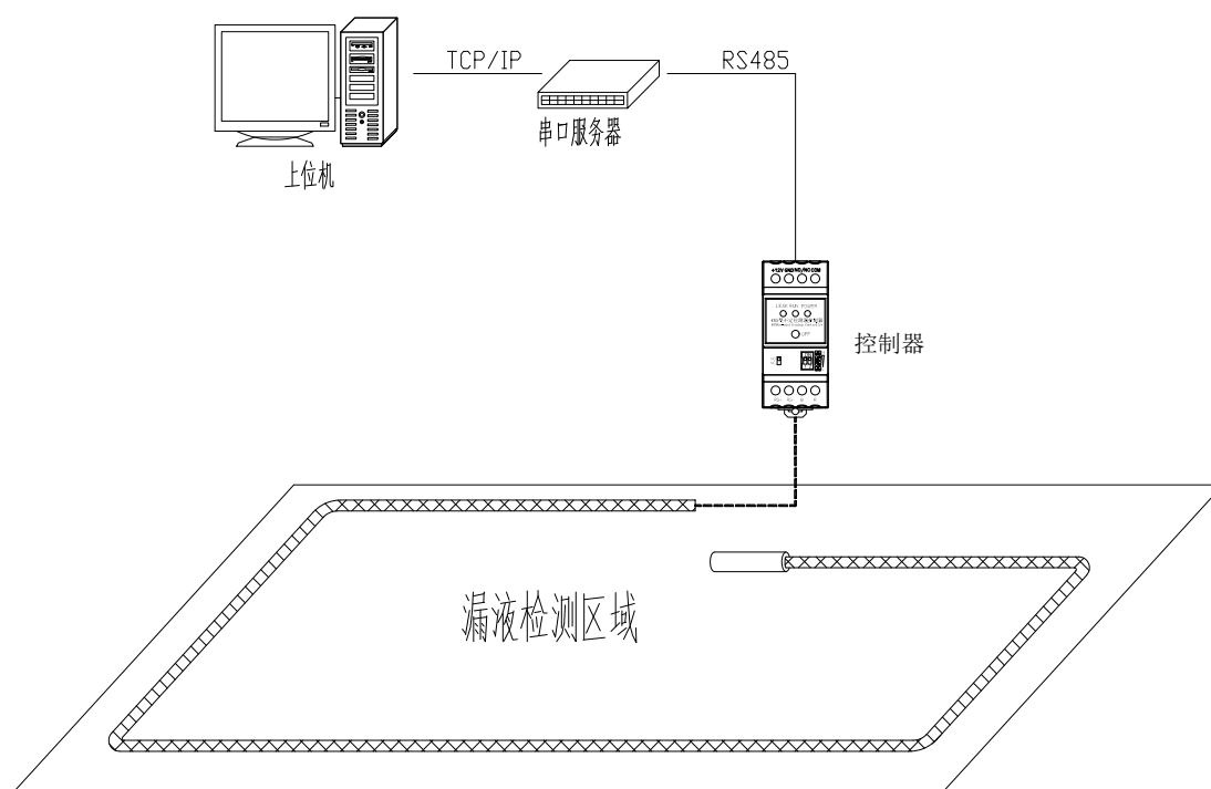
图 5 系统拓扑图
