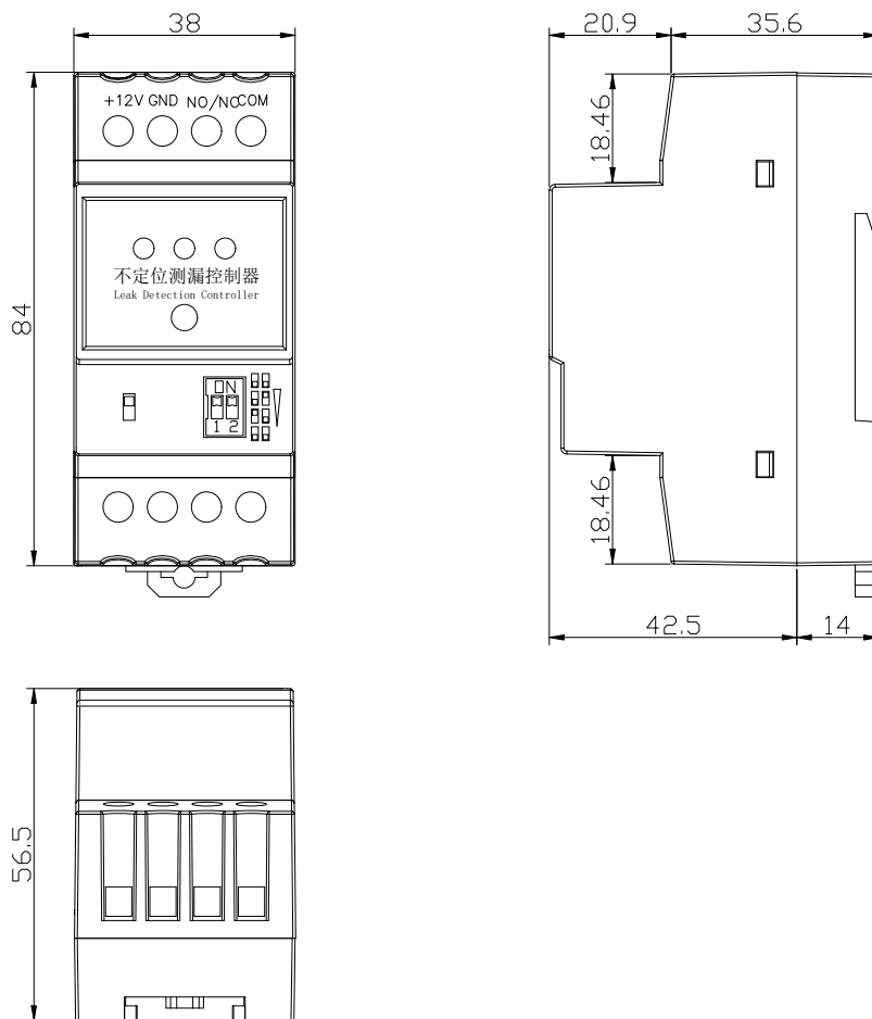
图 1 尺寸图
