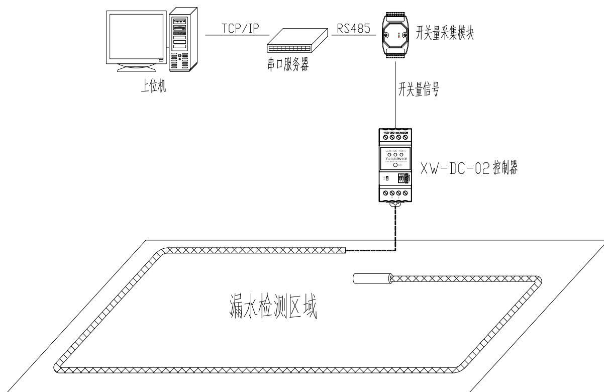
图 4 系统拓扑图
