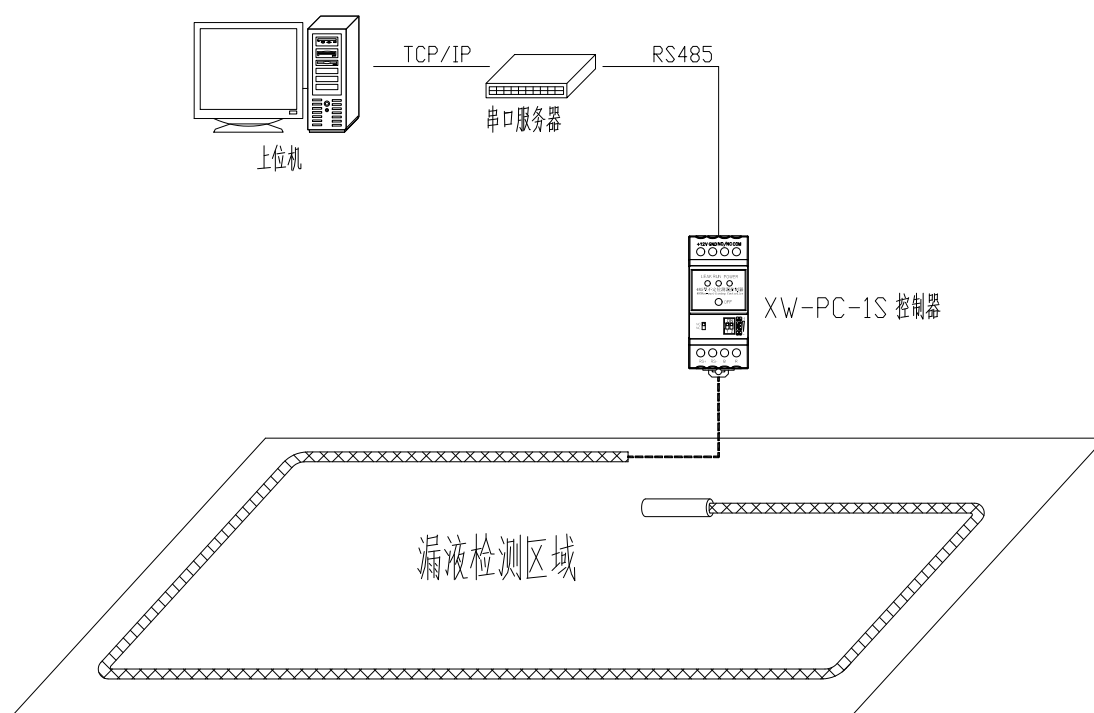
图 4 系统拓扑图
