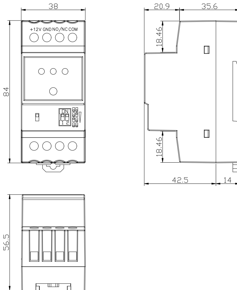
图 1 尺寸图
